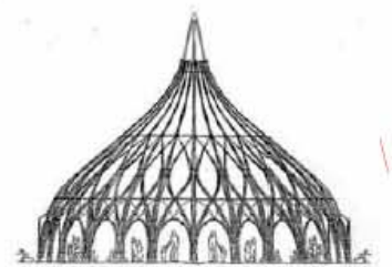
Ansicht M = 1: 100
